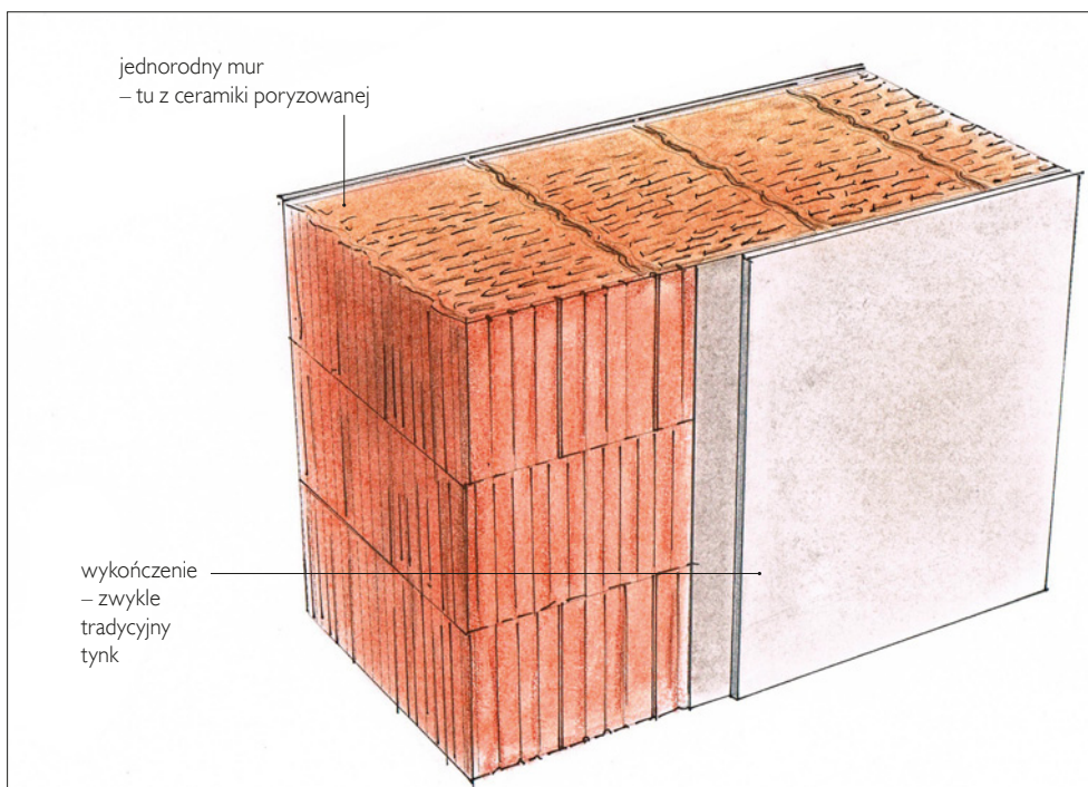
Ściana jednowarstwowa.
