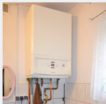
❶ Kompaktowy kocioł ma wbudowany zasobnik c.w.u. o pojemności 45 l.
