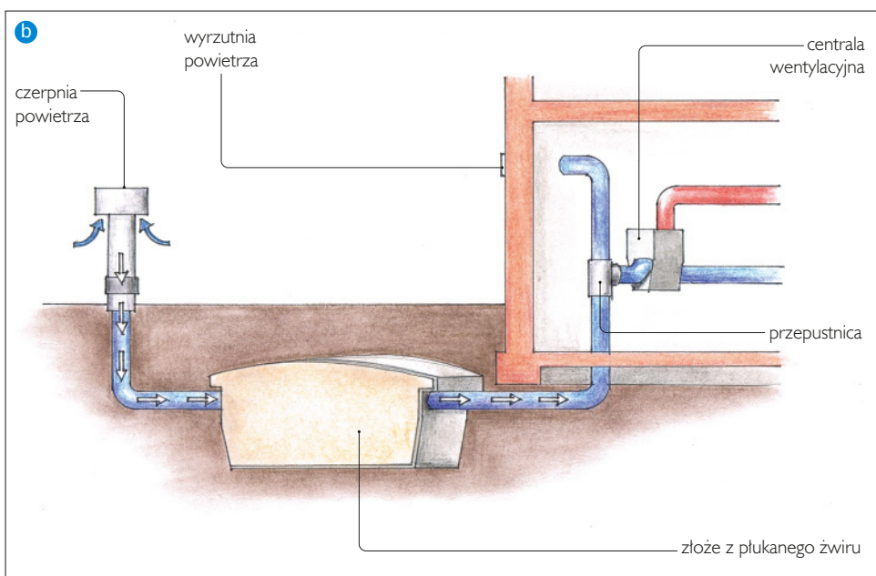
Gruntowy wymiennik ciepła rurowy (a), żwirowy (b).
