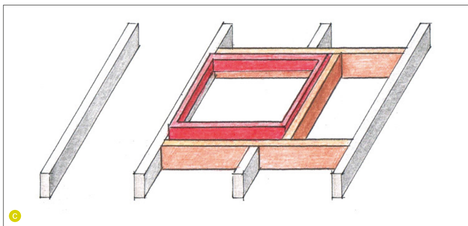
Montaż okna dachowego na krokwiach (a), łatach (b), wymianach (c).
