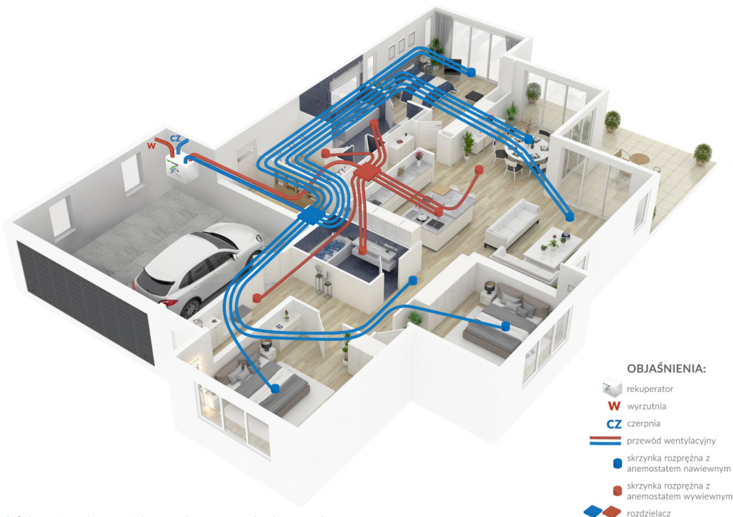
Schemat instalacji wentylacji mechanicznej z odzyskiem ciepła. TOPVAC
