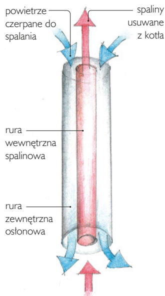
➔ Budowa systemu powietrzno-spalinowego.
