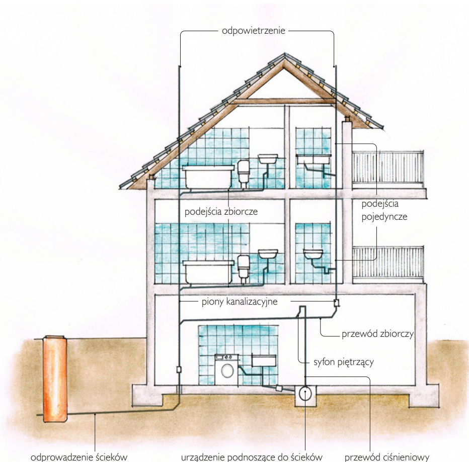
➔ Schemat domowej instalacji kanalizacyjnej.
