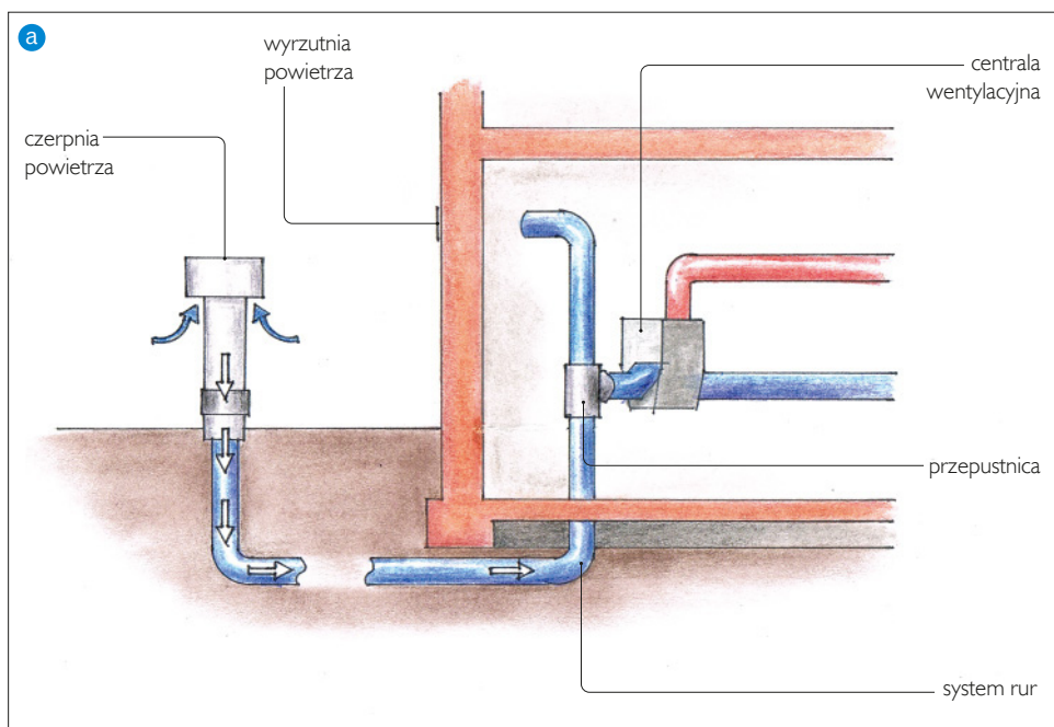
Czerpnia powietrza gruntowego wymiennika ciepła. PRO-VENT
