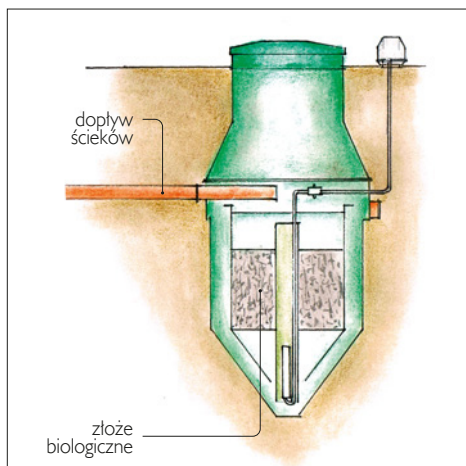
🔗 Oczyszczalnia ze złożem biologicznym.
