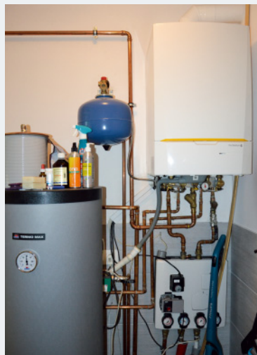
📌 Urządzenia grzewcze umieszczono w kotłowni o powierzchni 15 m 2 .
