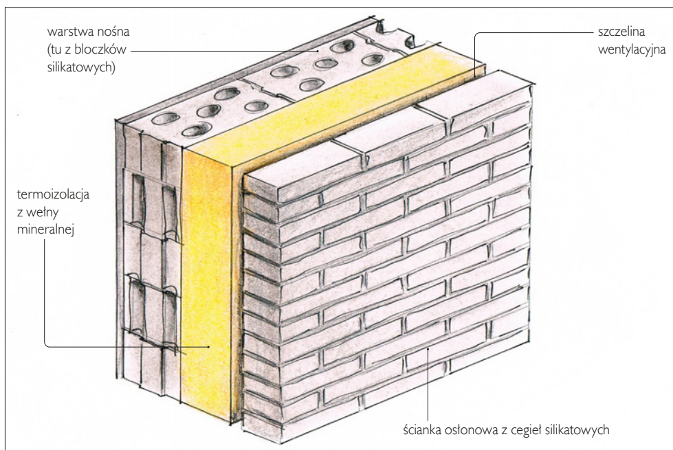
❶ Ściana trójwarstwowa.
