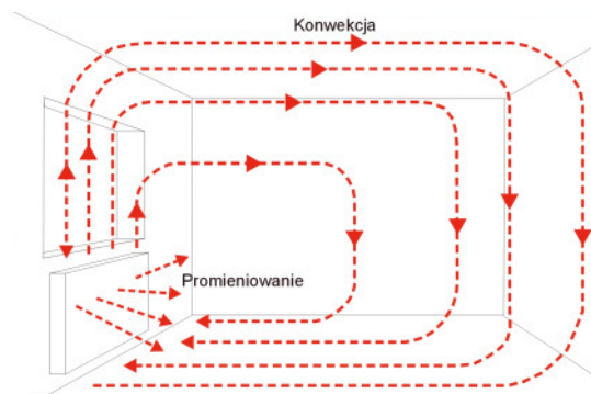
❶ Sposoby oddawania ciepła przez grzejnik ścienny.
