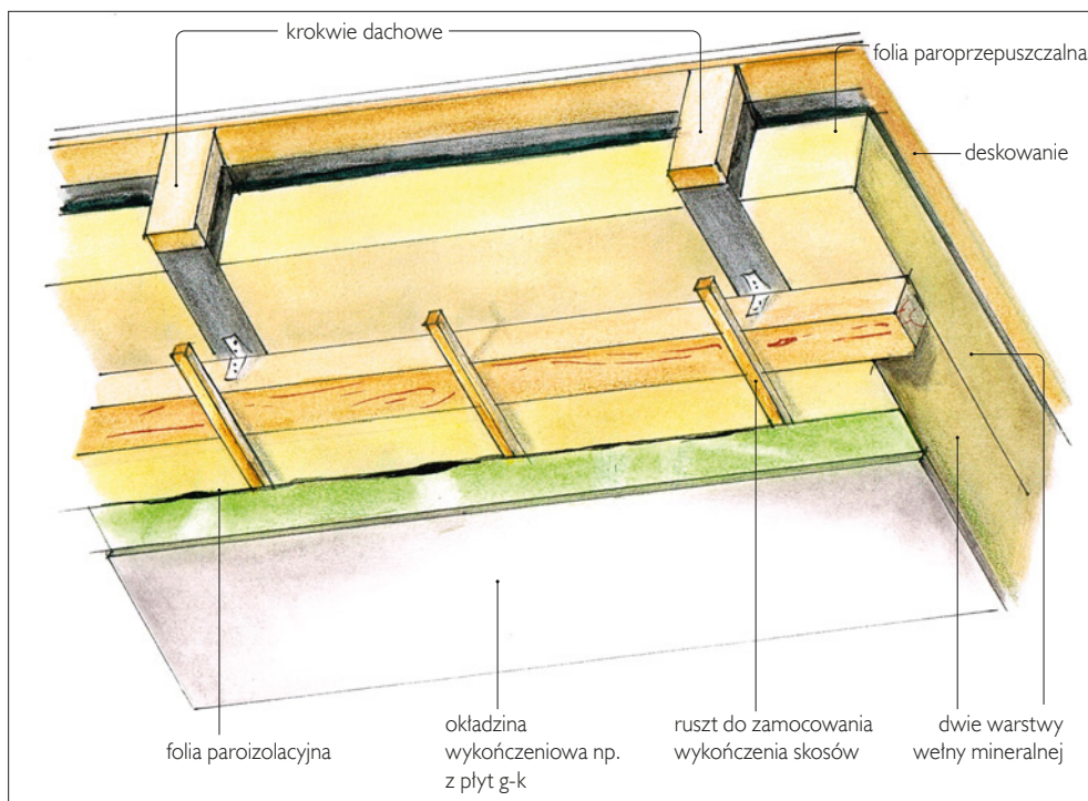
❶ Schemat ocieplenia dachu skośnego wełną mineralną.
