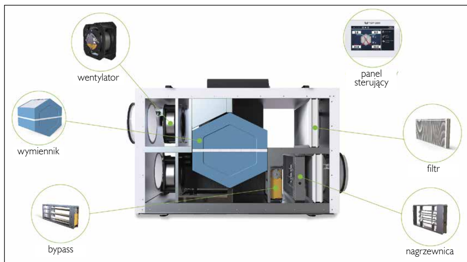
Centrała wentylacyjna z rekuperatorem. TOPVAC
