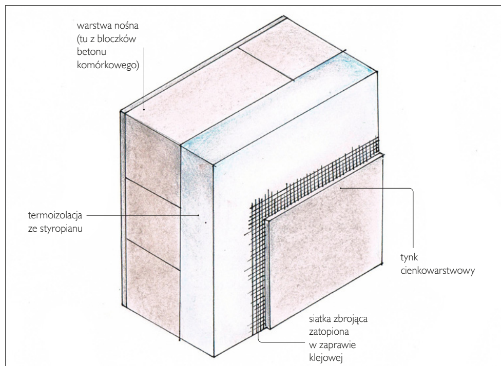
Ściana dwuwarstwowa ocieplona metodą lekką moką.
