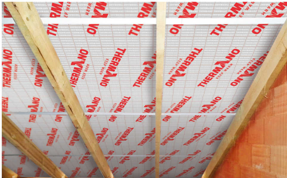
◄ Z wytrzymałych i odpornych na wilgoć płyt można ułożyć tzw. izolację nakrokwiową. THERMANO
