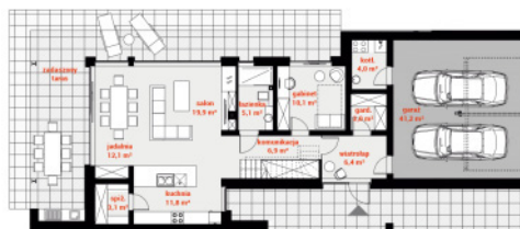
RZUT PARTERU
