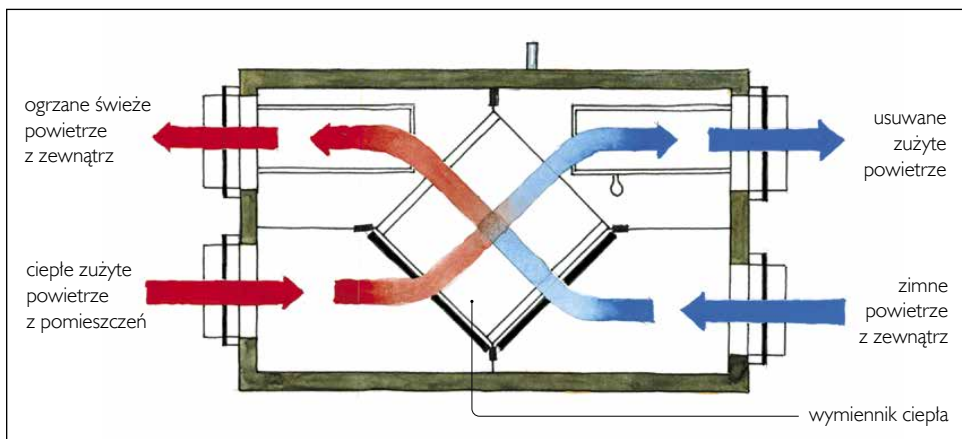
Schemat wymiany powietrza zużytego wywiewanego z rekuperatora i świeżego nawiewanego z zewnątrz.
