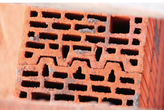
🔧 Przy murowaniu pustaków ze ściankami ukształtowanymi na pióro i wpust, w spoinach pionowych nie daje się zaprawy. J. WERNER
